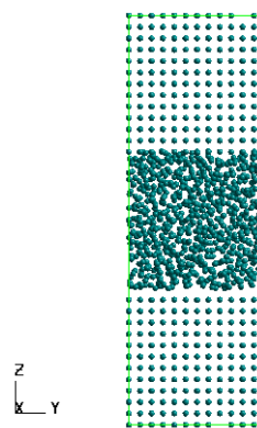
図.2 SLS 構造の初期配置
