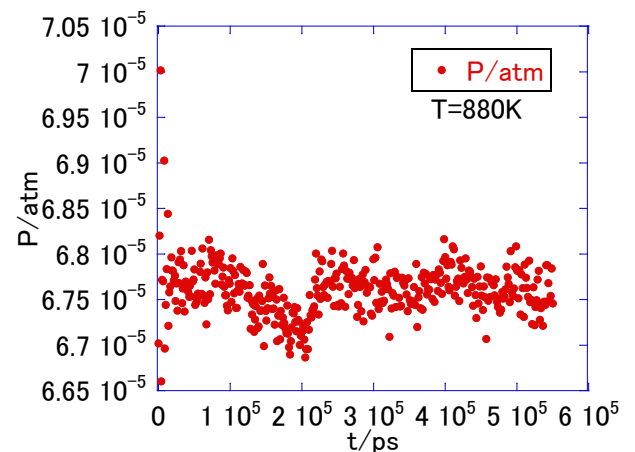
図.5 SLS 構造の初期配置から出発した場合の圧力の時間経過
