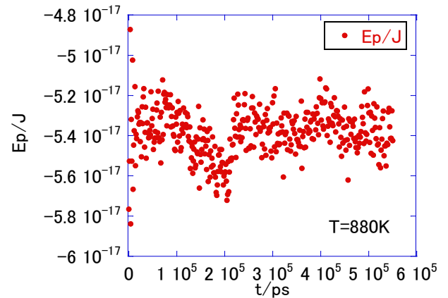
図.4 SLS 構造の初期配置から出発した場合のポテンシャルエネルギーの時間経過
