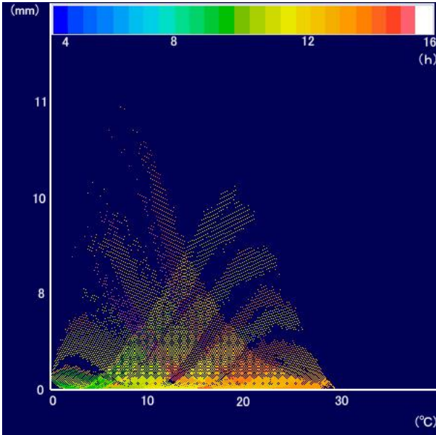
図 2 月平均気温と回帰式 (1) による月可能蒸発散量の差の分布
