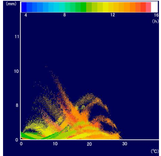
図 3 月平均気温と回帰式 (2) による月可能蒸発散量の差の分布
