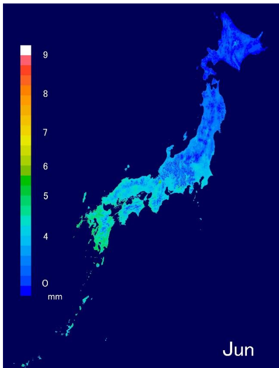
図 4 6 月の回帰式 (2) と月可能蒸発散量の差の分布図
