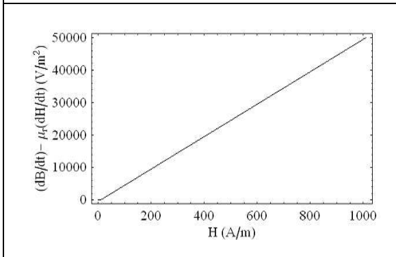
Fig.3 Hysteresis Parameter s (TDK H5A)
