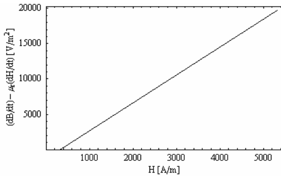
Fig. 3. Hysteresis parameter s (soft iron)
