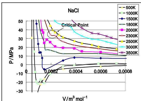
図 8. NaCl の圧力等温線
