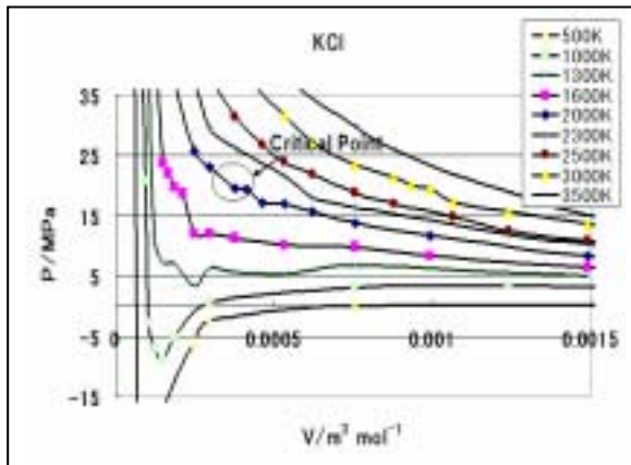
図 6. KCl の圧力等温線
