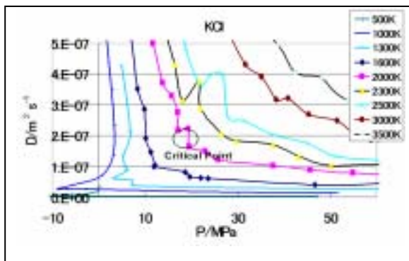
図 7. KCl の自己拡散係数の圧力依存性
