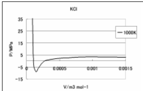
図 2. KCl 1000K の圧力等温線
