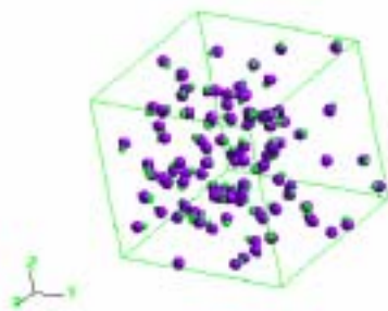
図 3. KCl 1000K 1MPa での分子配置
