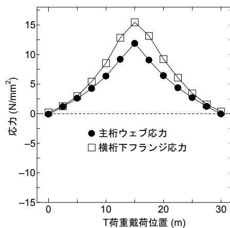
図 7. T 荷重による応力変動
