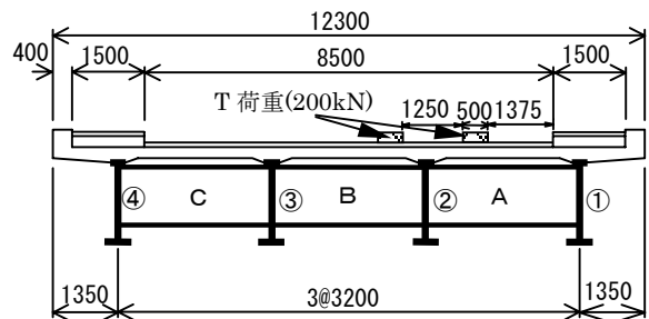
図 2. 設計断面 (単位: mm)
