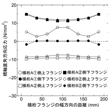
図 6. 横桁フランジの応力分布
