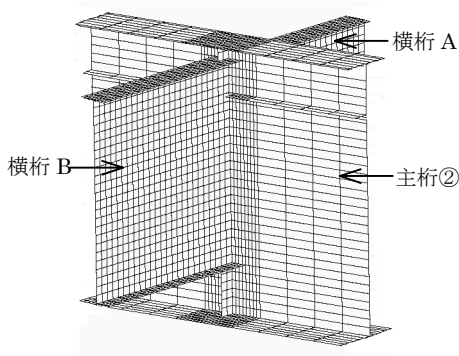
図 4. 主桁・横桁交差部の要素分割図
