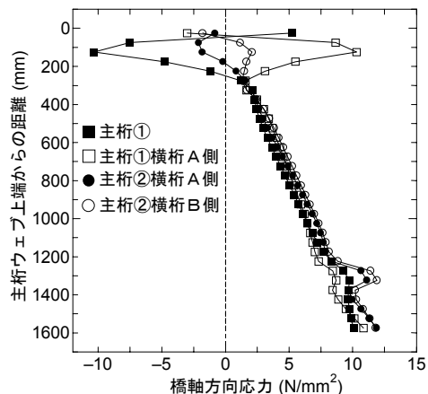
図 5. 主桁ウェブの応力分布
