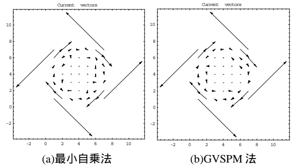
図4. 推定された電流分布
