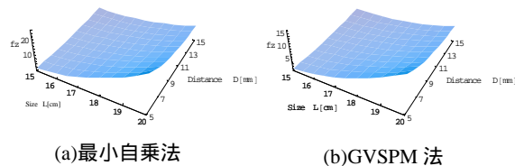
図3. 評価関数 f_z の変化
