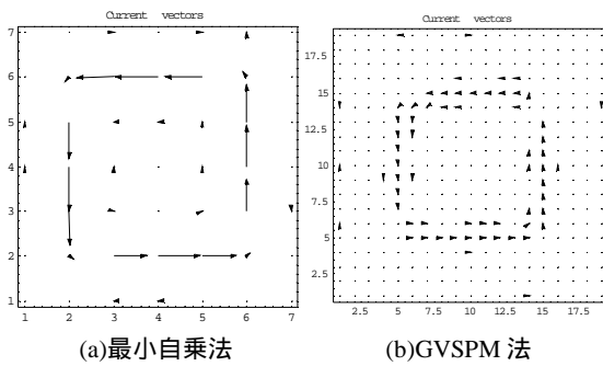
図 9. 畳み込み演算によって抽出された主要電流分布
