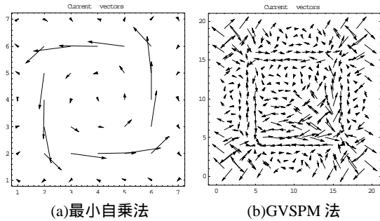
図 8. 推定された電流分布
