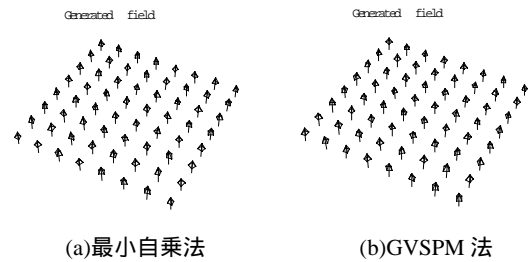
図5. 推定された電流分布が生成する磁界分布
