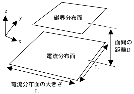
図1. 磁界分布制御装置のモデル
