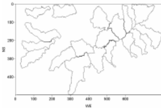
図8 流域の抽出結果
