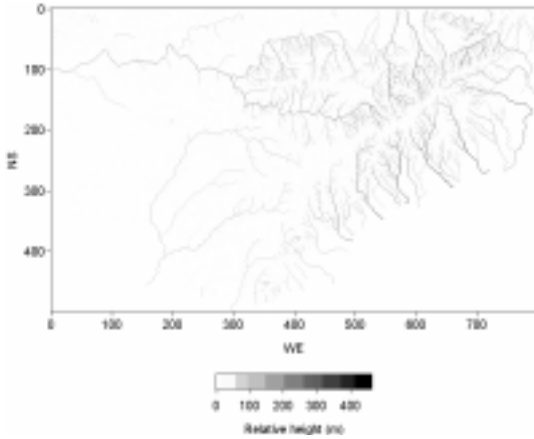
図6 流域平均比高の計算結果
