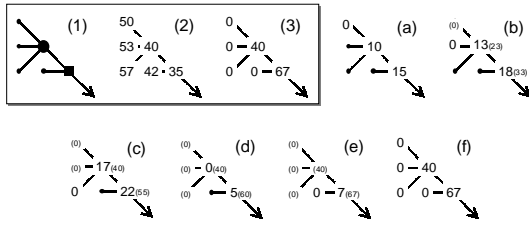
図5 山体体積の計算アルゴリズム
